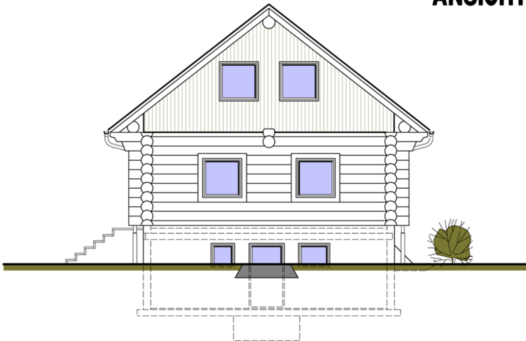
ANSICHT VON WESTEN
